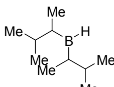
Disiamil borano
